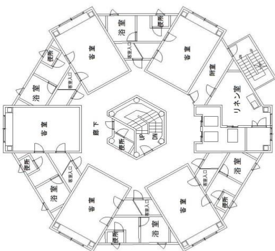
2~5階平面図
