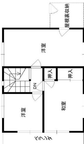
2階 平面図
