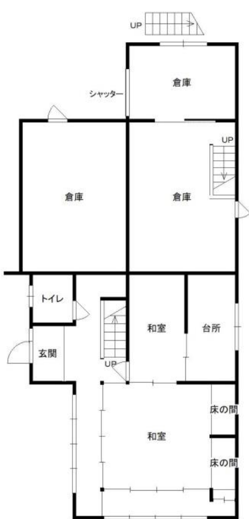
1階 平面図
