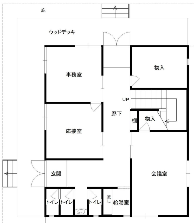
1階 平面図 附属建物 符号2
